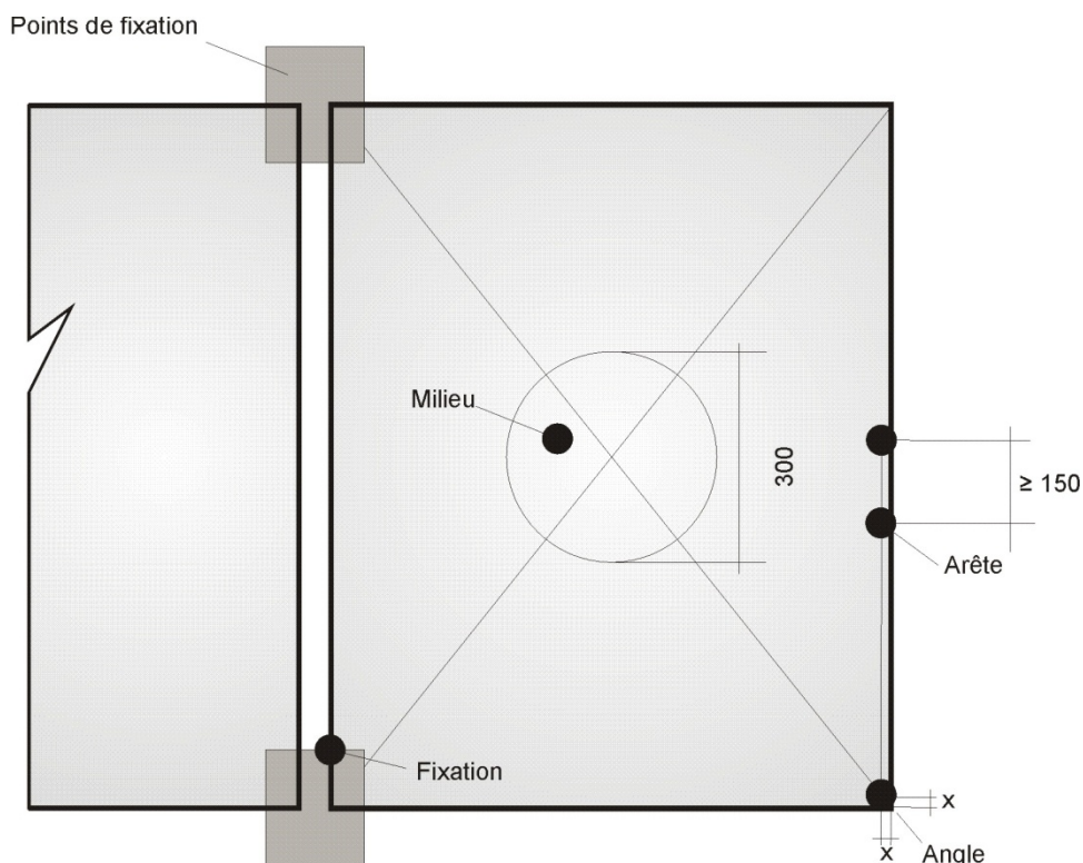
Figure 1 Points d'impact sur un vitrage de façade, vus en plan, à l'exemple d'un vitrage pourvu d'éléments de fixation extérieurs ( x = 1/5 du diamètre du projectile; dimensions en millimètres).
