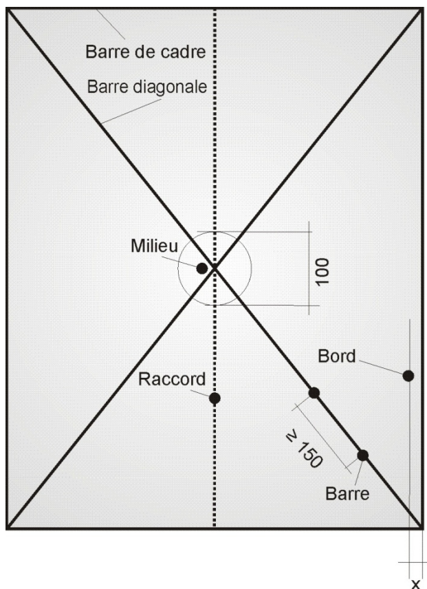
Figure 1 Points d'impact sur une construction assimilable à une tente, vue en plan ( x = 1/2 diamètre du projectile; dimensions en millimètres).
