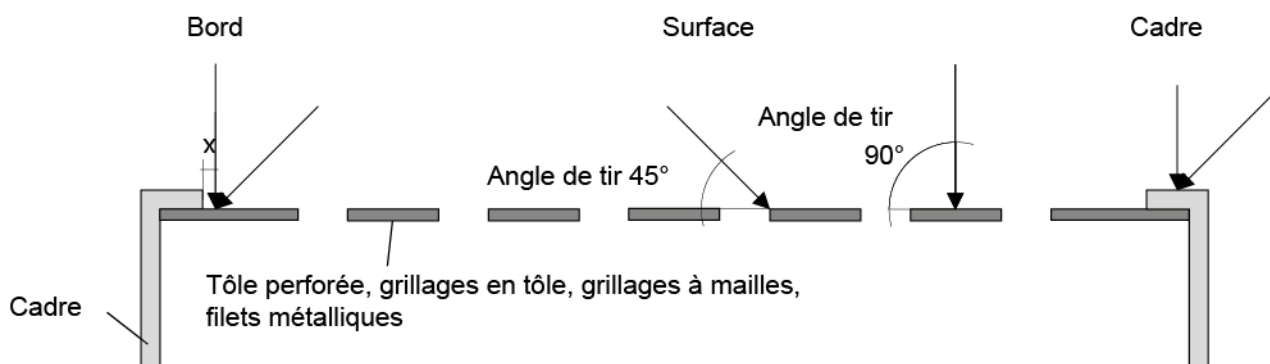
Illustration 5 : coupe, schématique
