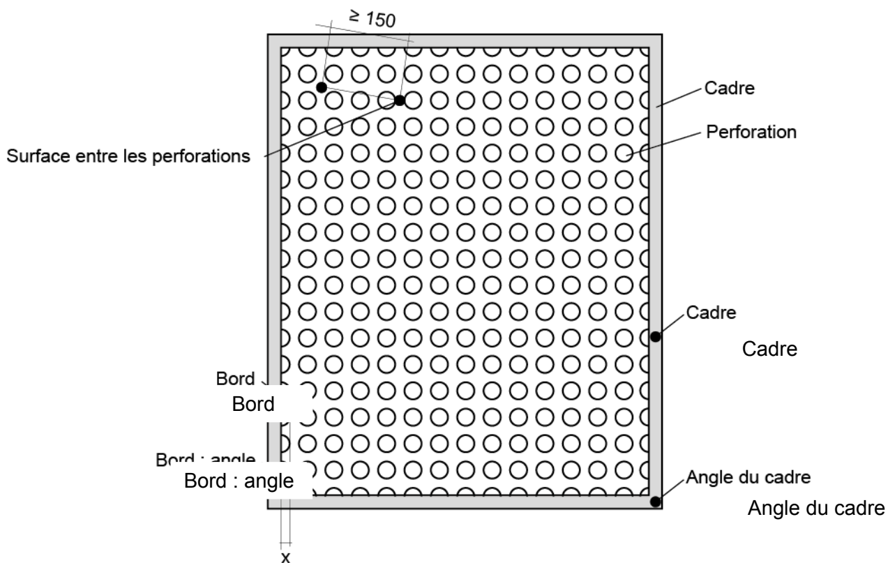
Illustration 3 : points d'impact vus en plan pour la tôle perforée ( x : 1/5 du diamètre du projectile, mesures en millimètres)
