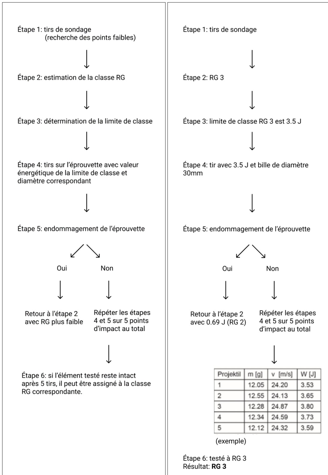
Figure 3 Schéma (à gauche) et exemple (à droite) du déroulement de l'essai.
