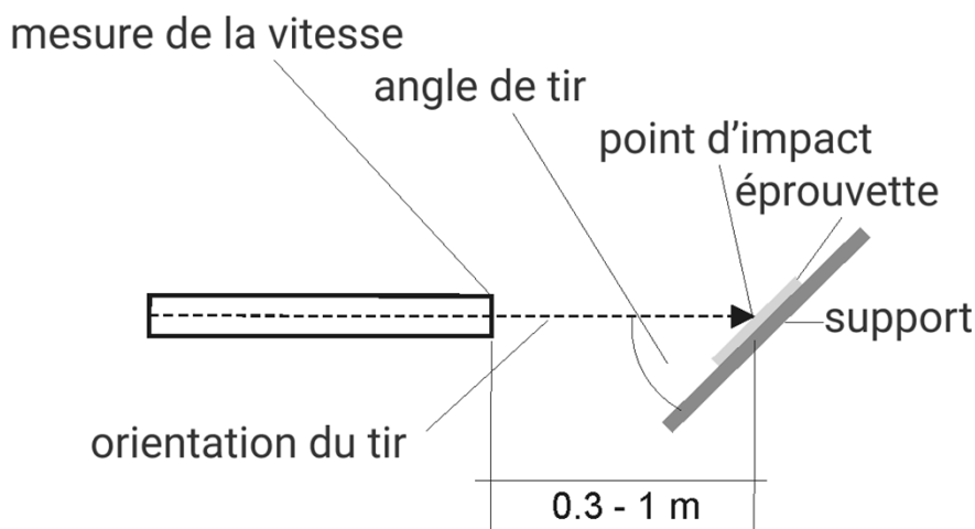
Figure 1 Appareillage configuré pour simuler l'impact d'un grêlon tiré en direction horizontale sous un angle de 45^\circ \pm 2^\circ (dimensions en mètres).
