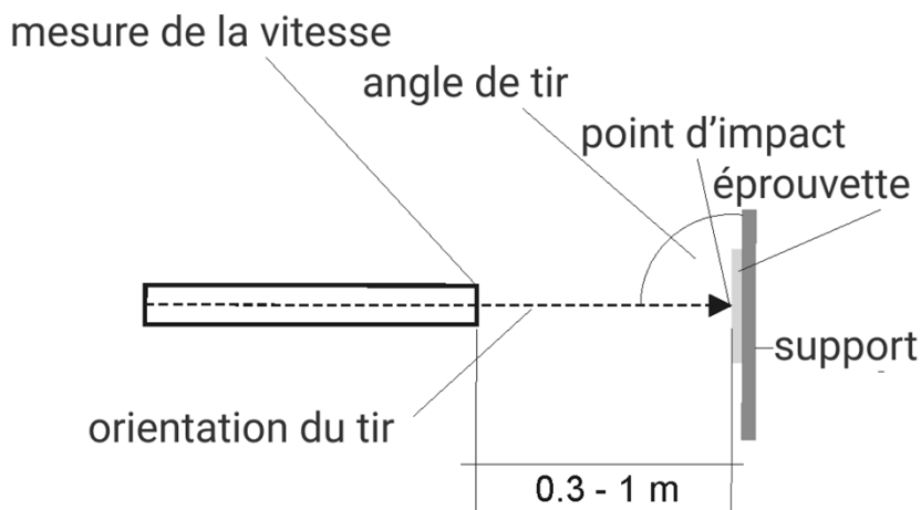
Figure 2 Appareillage configuré pour simuler l'impact d'un grêlon tiré en direction horizontale sous un angle de 90^\circ \pm 2^\circ (dimensions en mètres).
