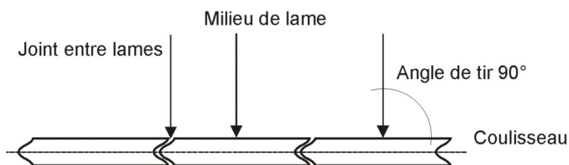
Figure 4 Points d'impact et angle de tir pour un volet roulant destiné à un toit, vus en coupe.
