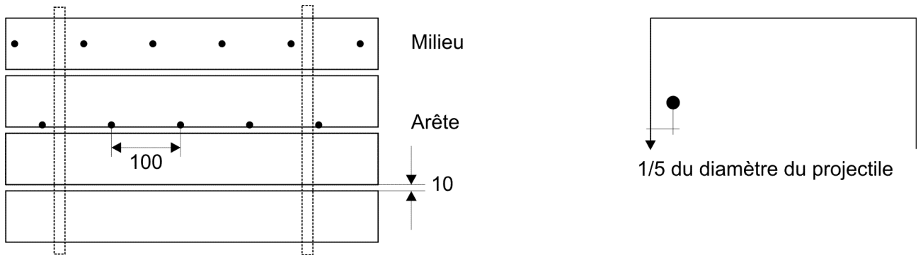
Figure 1 Points d'impact sur des éléments en bois, vus en plan (dimensions en millimètres)
