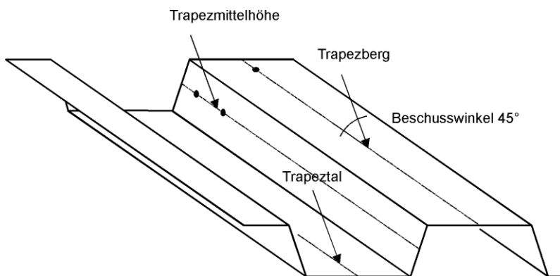
Abbildung 6 Besussorte und Besusswinkel bei selbsttragenden Profilen mit vertikaler Ausrichtung des Profils, hier am Beispiel des Trapezblechs
