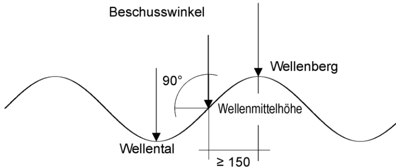
Abbildung 5 Besussorte und Besusswinkel des profilierten Blechs als Dachbauteil im Seitenriss, hier am Beispiel des Wellblechs (Masse in Millimeter)
