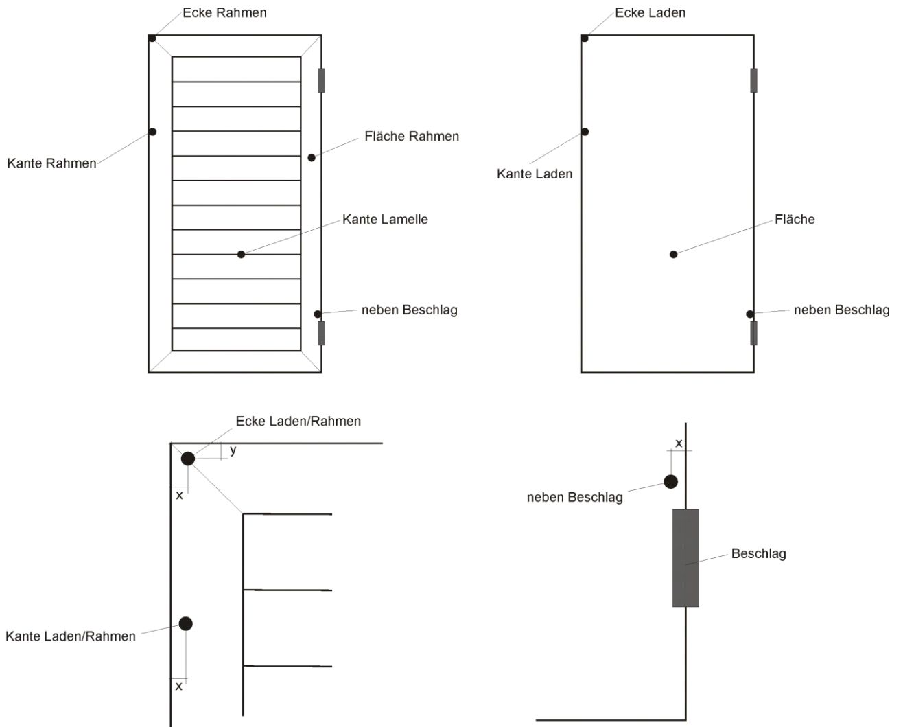
Abbildung 1 Beschussorte am Beispiel eines gerahmten Drehladens mit Lamellen (oben links) und am Beispiel eines ungerahmten Drehladens ohne Lamellen (oben rechts). Unten links und rechts befinden sich Detailskizzen der Beschussorte Ecke Laden/Rahmen, Kante Laden/Rahmen und Kanten neben dem Beschlag; x und y entsprechen 1/5 Projektildurchmesser
