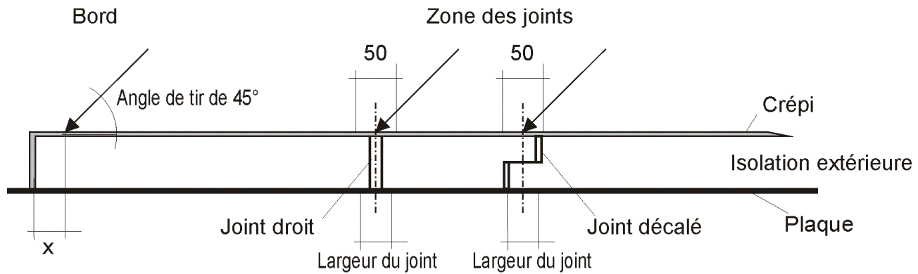
Figure 3 Vue de profil des points d'impact sur la zone des joints (à l'exemple d'un joint droit et d'un joint décalé) et sur le bord de l'échantillon ( x = 1/5 du diamètre du projectile, mesuré en millimètres)
