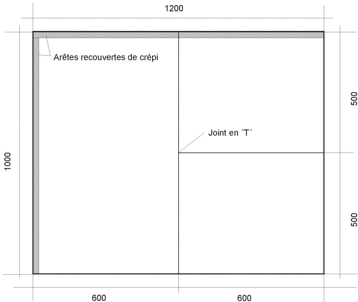
Figure 1 Configuration des essais de crépi, posé sur trois panneaux d'isolation extérieure (dimensions en millimètres)
