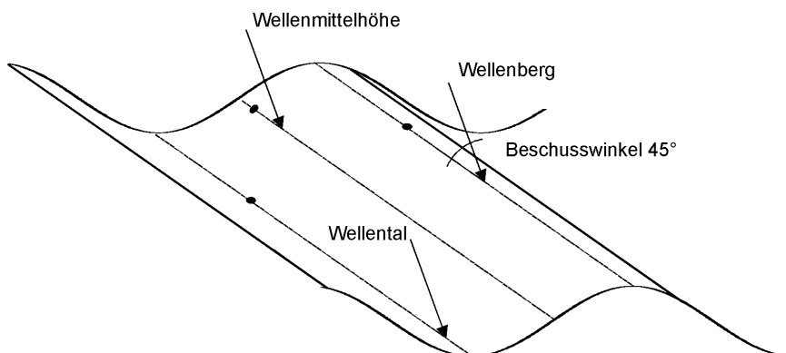
Abbildung 4 Beschussorte und Beschusswinkel der profilierten Bitumenplatte als Fassadenbauteil bei vertikaler Ausrichtung des Profils hier am Beispiel der gewellten Bitumenplatte
