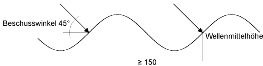
Abbildung 3 Beschussorte und Beschusswinkel der profilierten Bitumenplatte als Fassadenbauteil bei horizontaler oder diagonaler Ausrichtung des Profils hier am Beispiel der gewellten Bitumenplatte (Masse in Millimeter)
