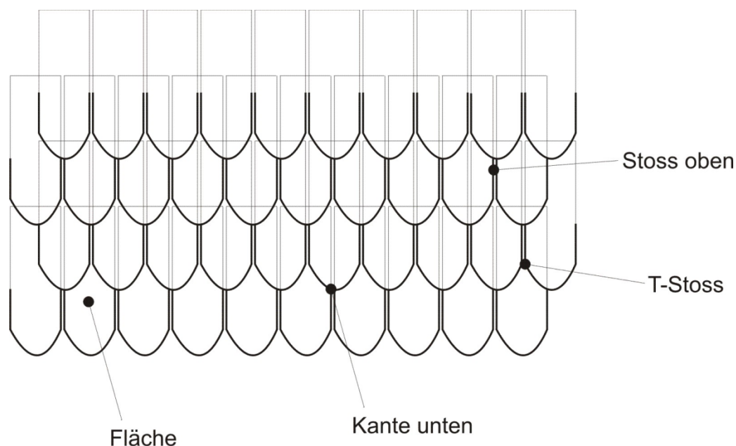
Abbildung 1 Beschussorte der Schindeln, Schindelform exemplarisch
